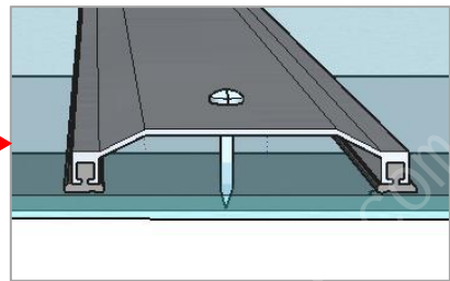
铝压条(6M/根)
