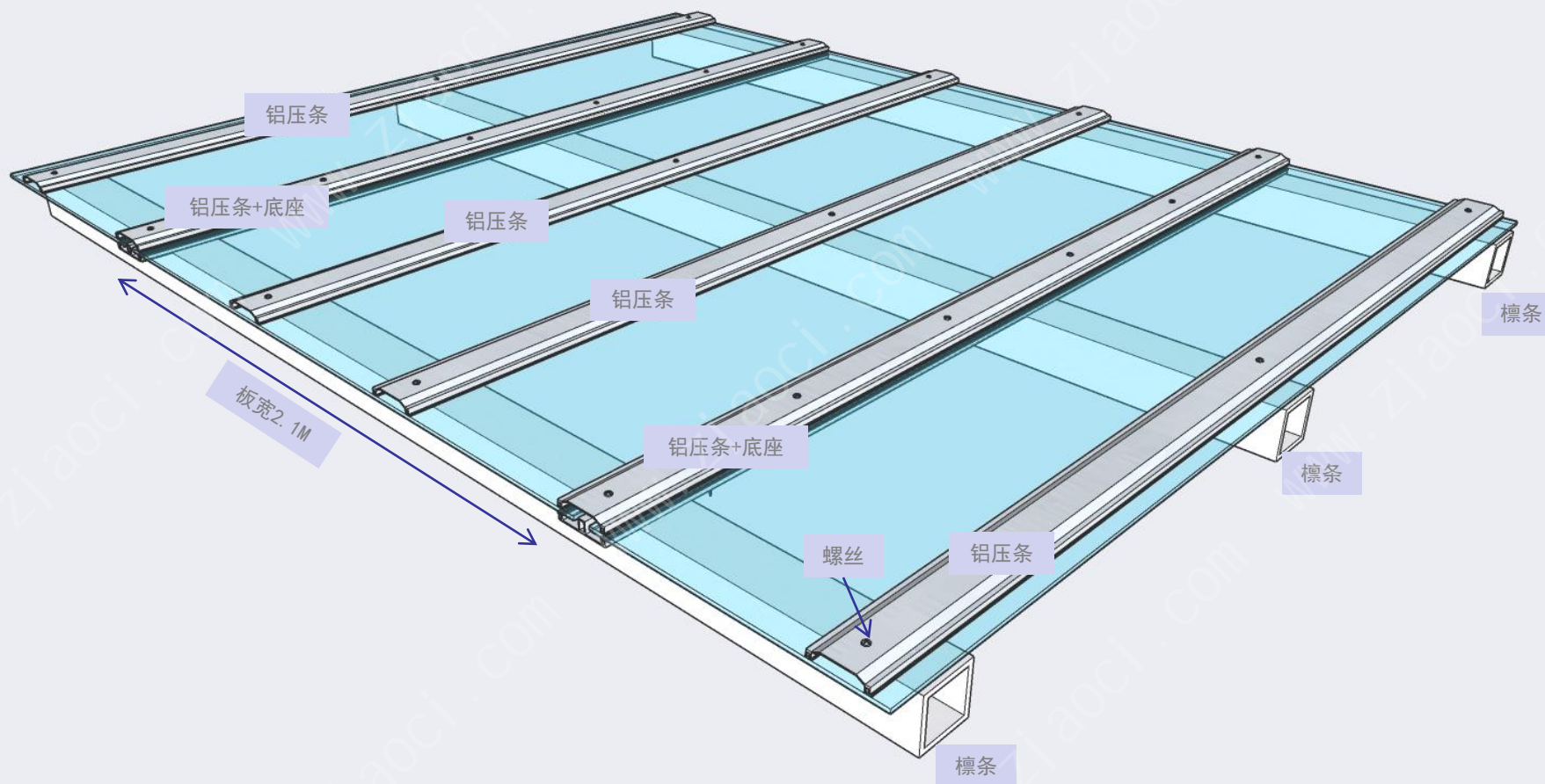
阳光板雨棚-结构图
