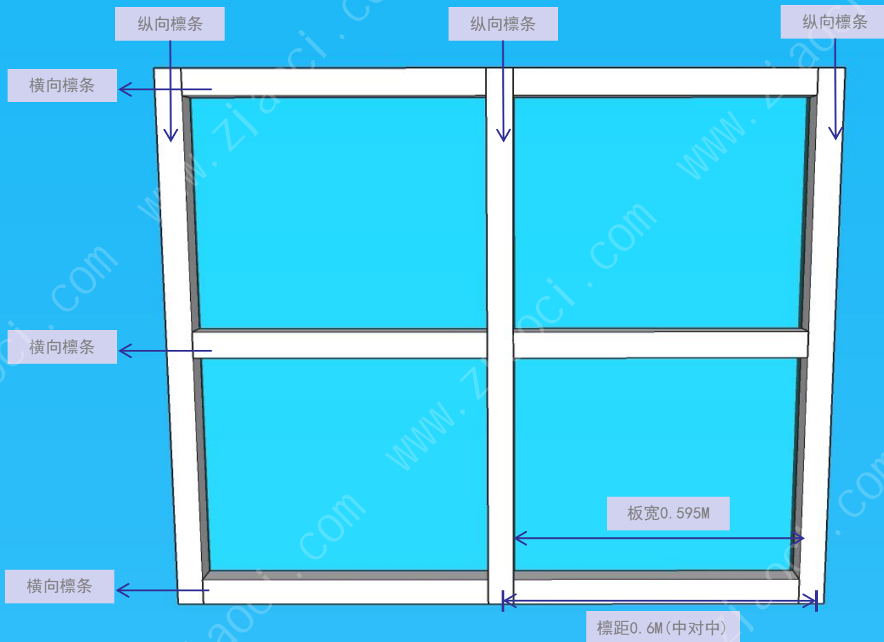
耐力板雨棚-仰视图
