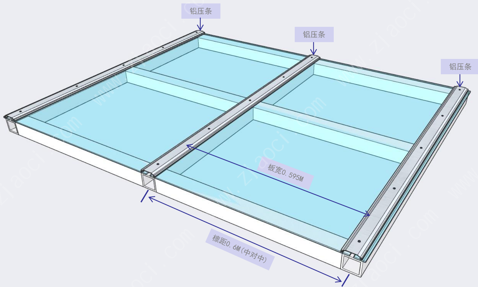
耐力板雨棚-结构图
