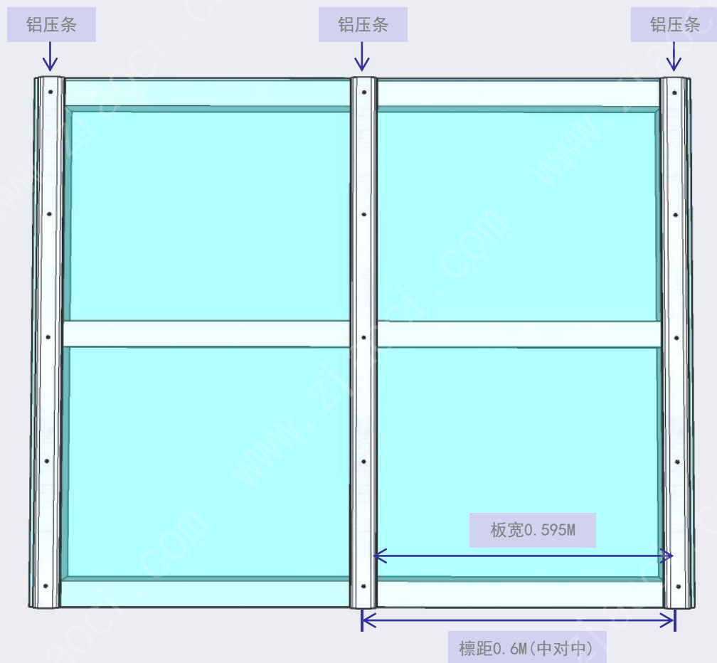
耐力板雨棚-俯视图
